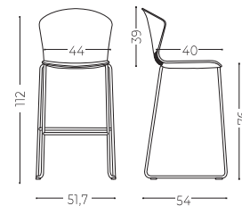
Cantilever stool Taburete Patin de acero
