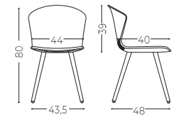
4 Wood legs chair Silla 4 patas de madera
