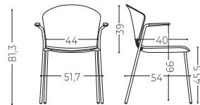
4 Metal legs chair Silla 4 patas de acero
