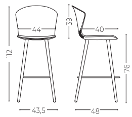
4 Wood legs stool Taburete 4 patas de madera
